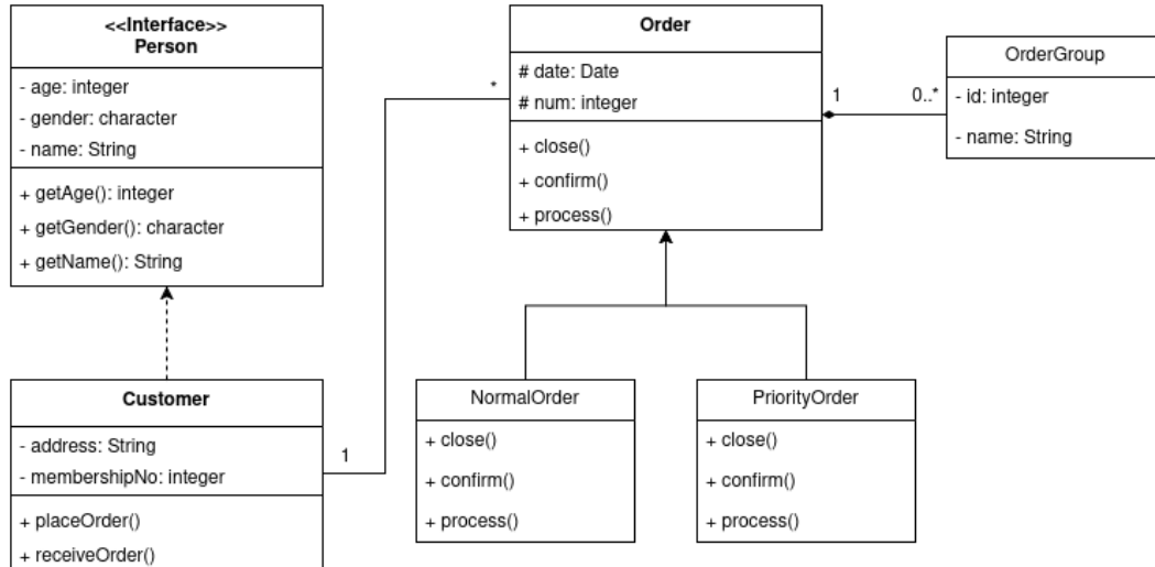
Figura 5.2: Esempio class diagram
