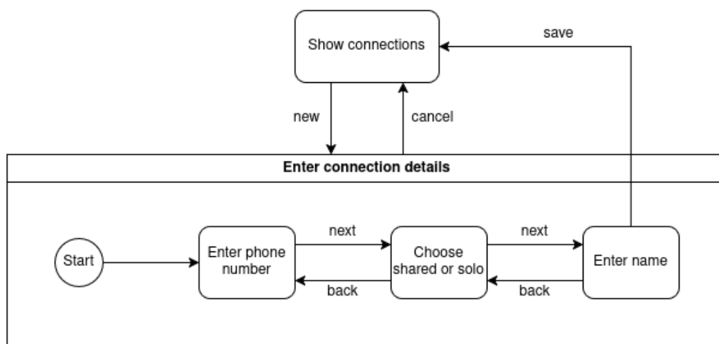
Figura 5.7: Esempio stato composito
